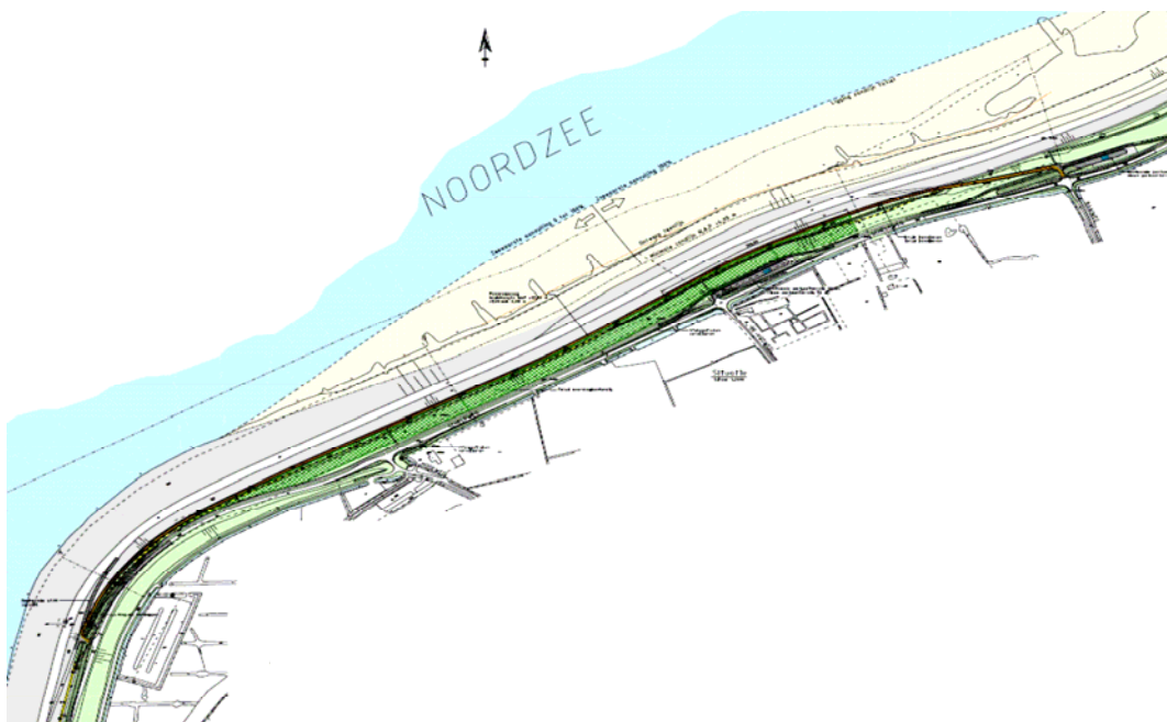
Figuur 1 Voorontwerp kustversterking zeedijk (opgesteld door WZE)
